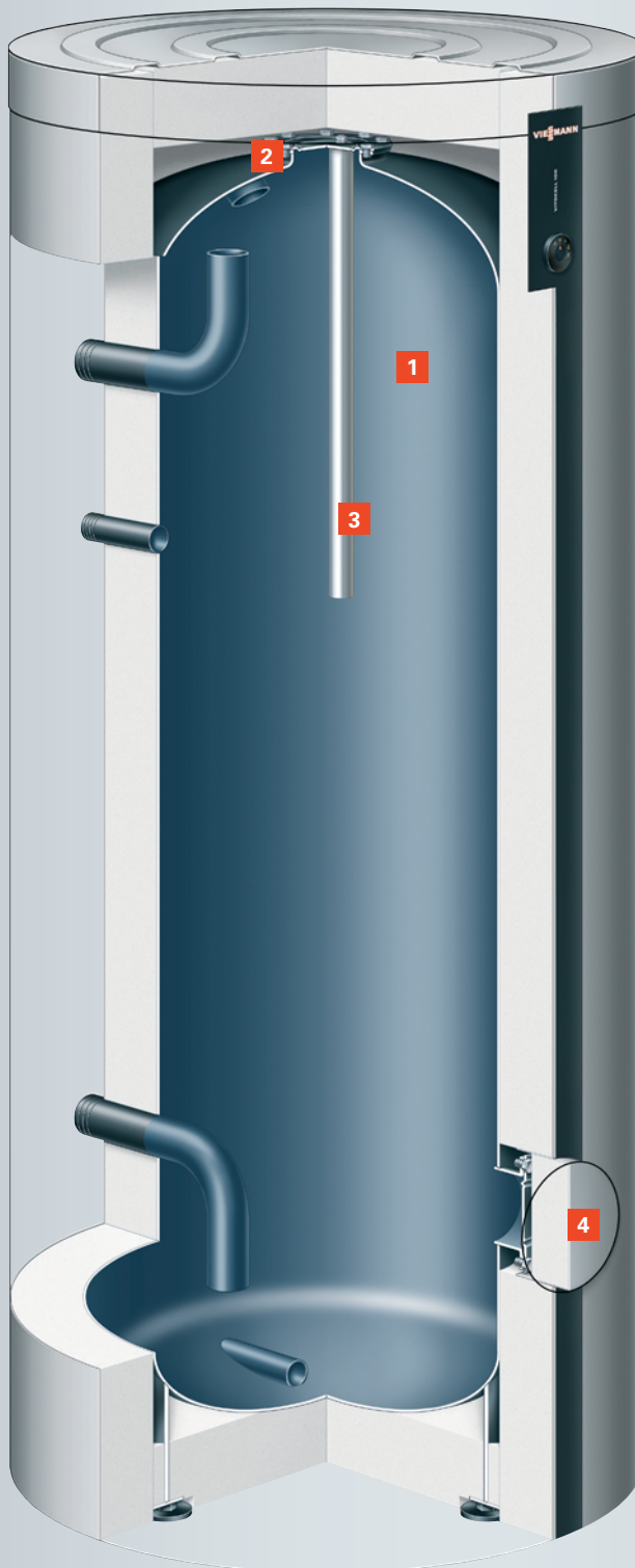
Vitocell 100-L (Typ CVL, 500 Liter Inhalt)
